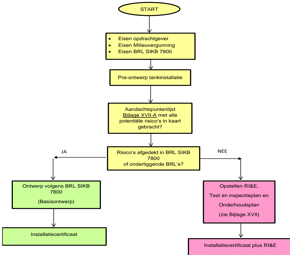
Figuur 7.1: Het ontwerp van een tankinstallatie
